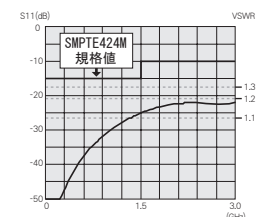
DCJ-LRのリターンロス
