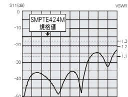
DCP-C25HDのリターンロス
