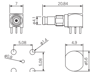
<プリント基板加工図> <取付穴寸法>
