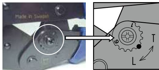
クリンプハイト調整ダイヤル
