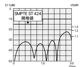
BCP-C6HDのリターンロス
