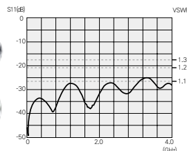
TNP-C3のリターンロス
