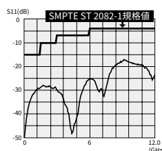
BCJ-BPLHK2Pのリターンロス
