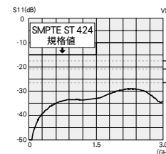
BCJ-BPLHAのリターンロス
