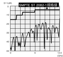
HBCP-D25HDAのリターンロス
