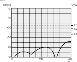
BJ-Jのリターンロス
