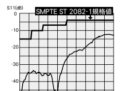
KCM-PCのリターンロス
