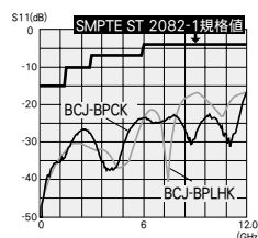
BCJ-BPCK BCJ-BPLHKのリターンロス
