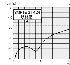
BCJ-BPC2Pのリターンロス
