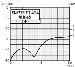
BCJ-BPLH2PAのリターンロス
