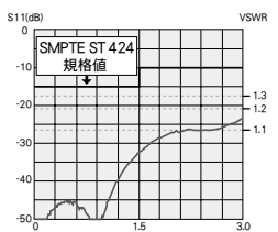
BCJ-FPLVAのリターンロス
