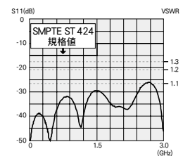
BCP-A3のリターンロス
