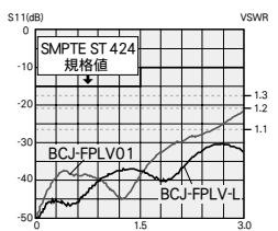
BCJ-FPLV01 BCJ-FPLV-Lのリターンロス
