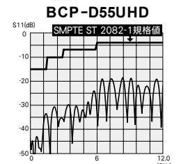
BCP-D55UHDのリターンロス
