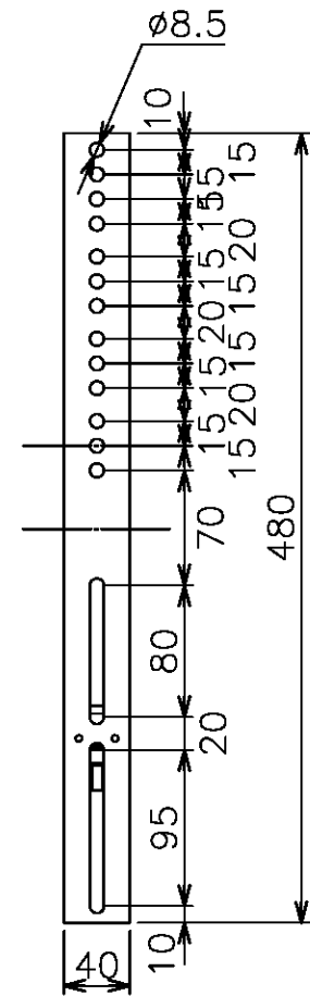
アタッチメント穴位置図
