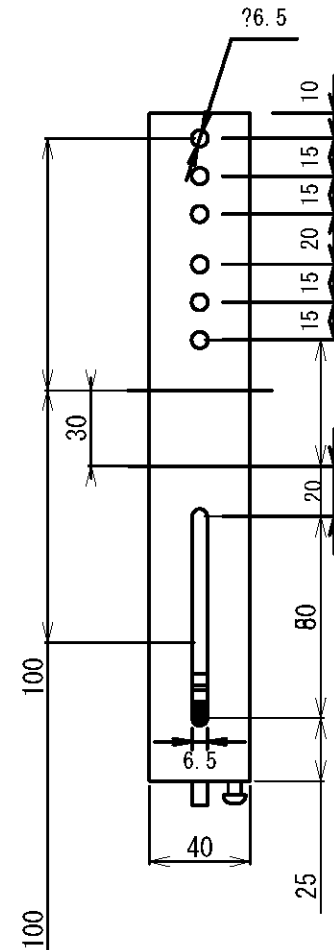
アタッチメント穴位置図
