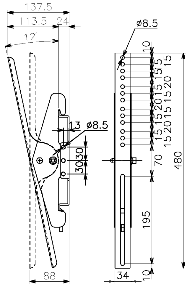
アタッチメント穴位置図
