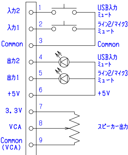
回路図
