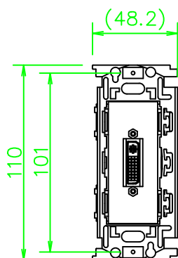
KP-DVIJ-*
