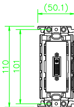
ZP-DVIJ-*
