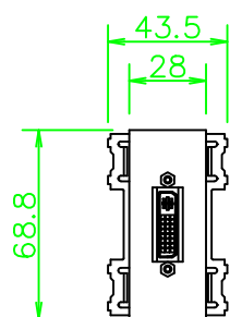
CP-DVIJ-*
