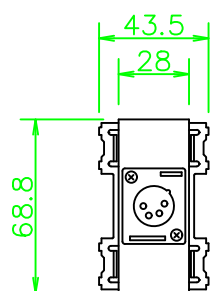
CP-4X2S-*
