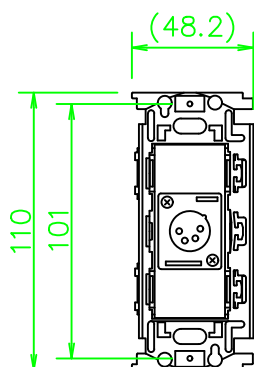
KP-4X2S-*
