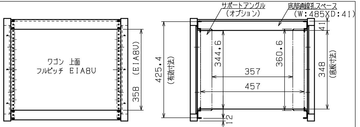
＜サポートアングル取合断面図＞
